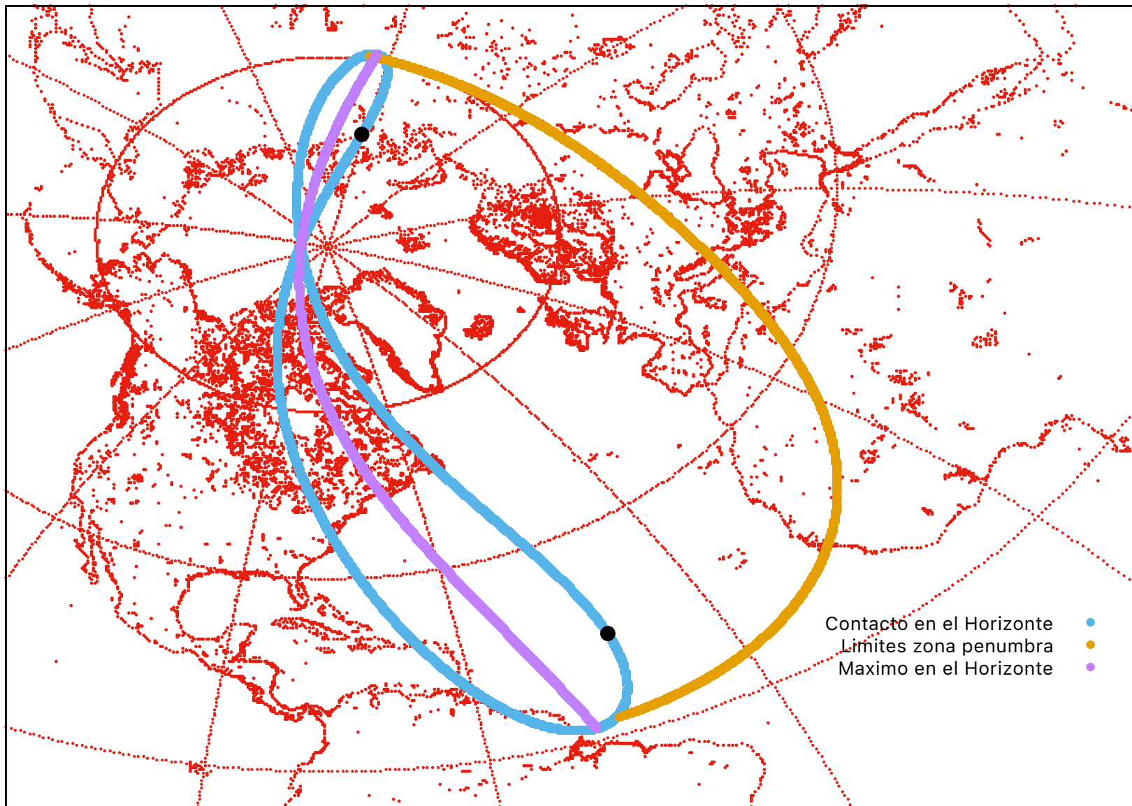
Eclipse 29 de marzo de 2025 (proy. estereografica)
