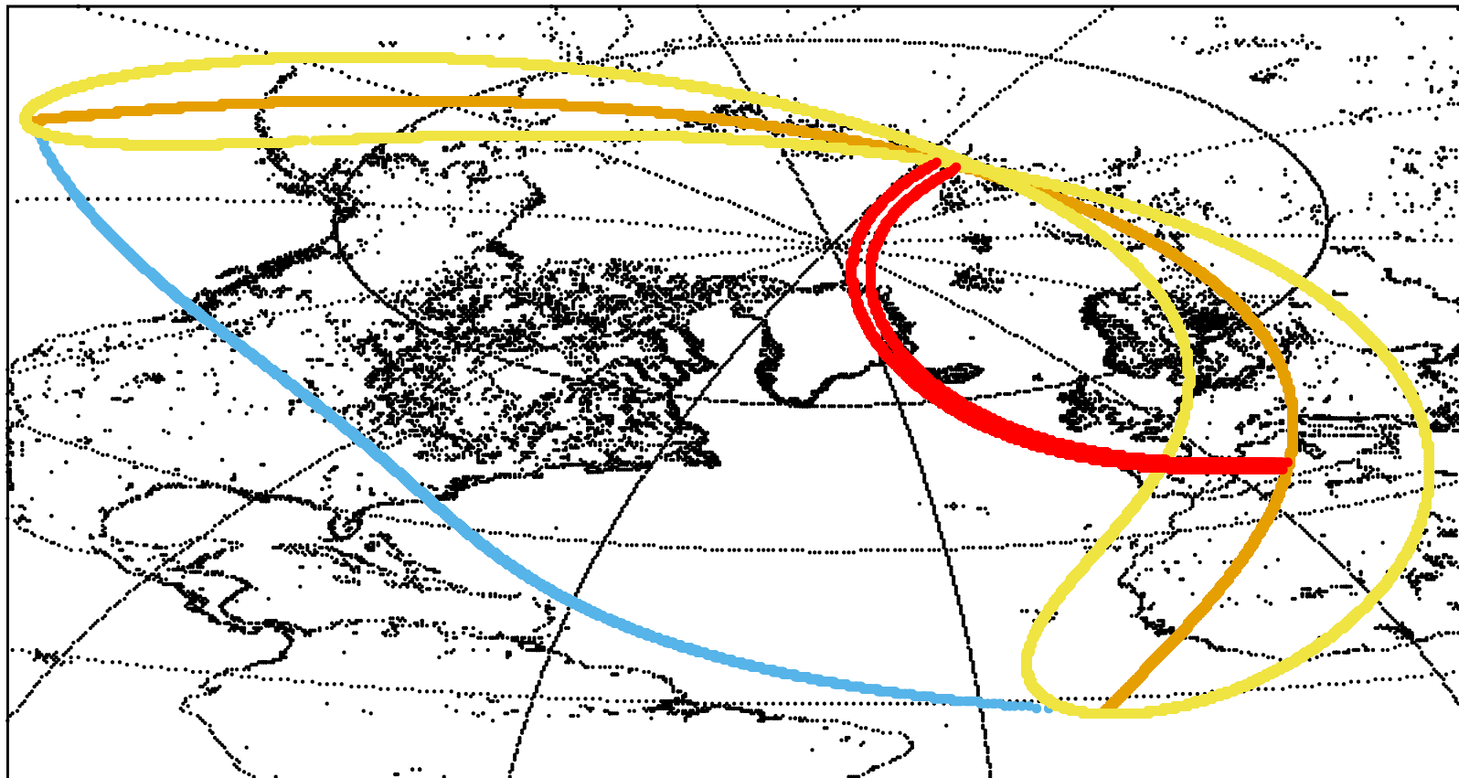
Eclipse 12 de Agosto de 2026 (Proy. Estereografica).
